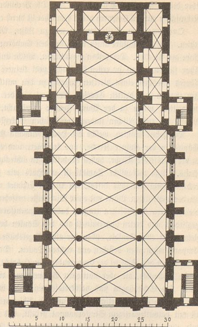
Bild 16. Paderborn. Kirche des hl. Franz Xaver. Grundriß.
