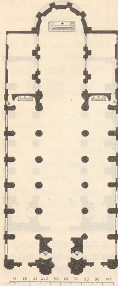
Bild 6. Köln. Idea II Bavarica. Grundriß.
