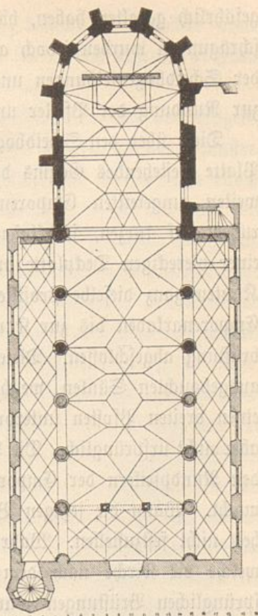
Bild 1. Koblenz. Grundriß 1 .
