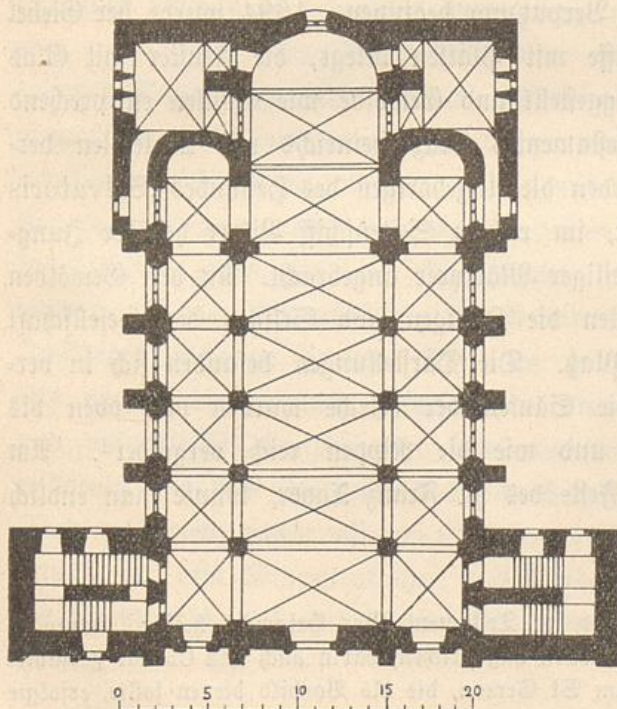
Bild 17. Bonn. Namen-Jesuitenkirche. Grundriß.
