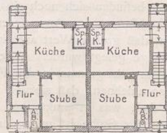
Abb. 7. Erdgeschoß.
