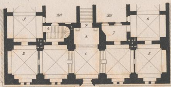
UNTERER GRUNDRISS
