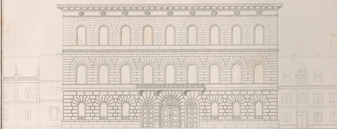
VORDER ANSICHT DES RATHHAUSES.
