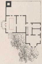
DAMPFMASCHINEN-HAUS.
