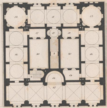
OBERER GRUNDRISS
