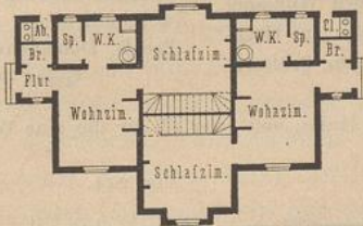
Erdgeschoß.
