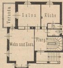
Einfamilienhaus zu Zürich.
