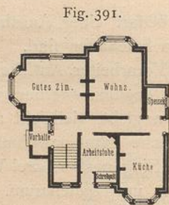
Fig. 391. Erdgeschoss.
