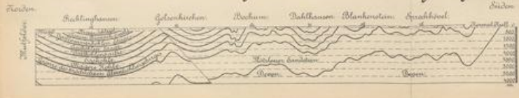
Schnitt durch das Westfälische Steinkohlengebirge.
