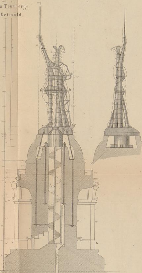
Querschnitt nach l m. mit dem Befestigungs Eisengerüste.
