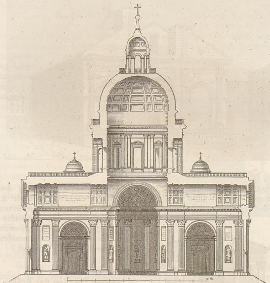
Fig. 51. Madonna da Carignano. Durchschnitt.
