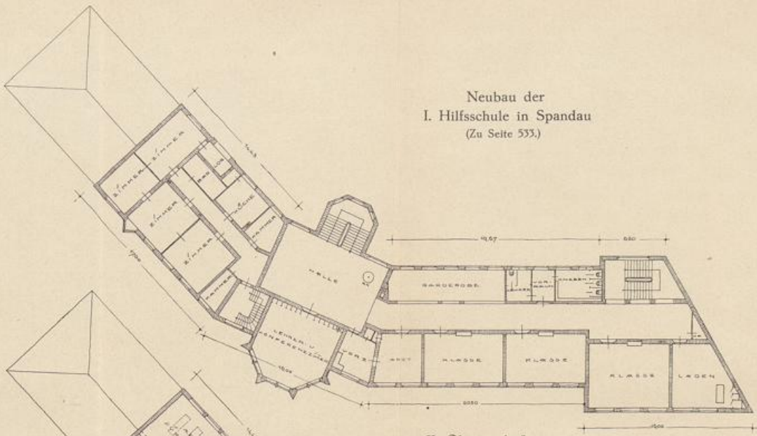
II. Obergeschoß
