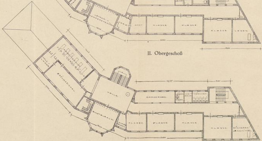
III. Geschoß
