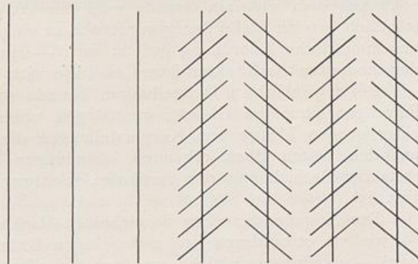
67. ZÖLLNERSCHE FIGUR.
