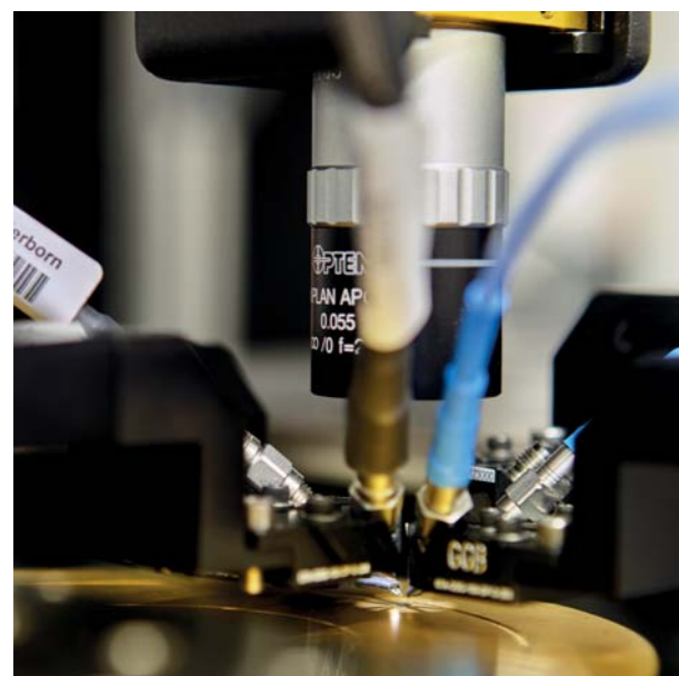
Aufbau zum HF-Test des gefertigten Chips RF test setup of the fabricated chip
