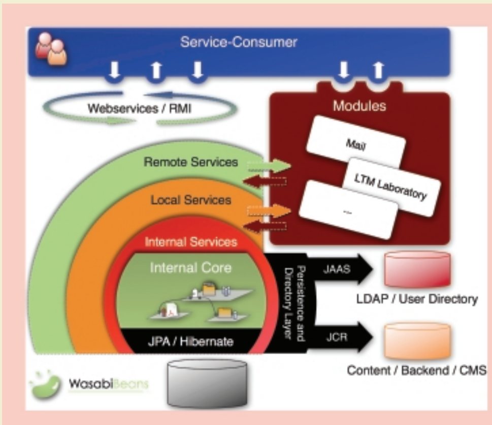
Abb. 5: Architektur des WasabiBeans-Frameworks.
