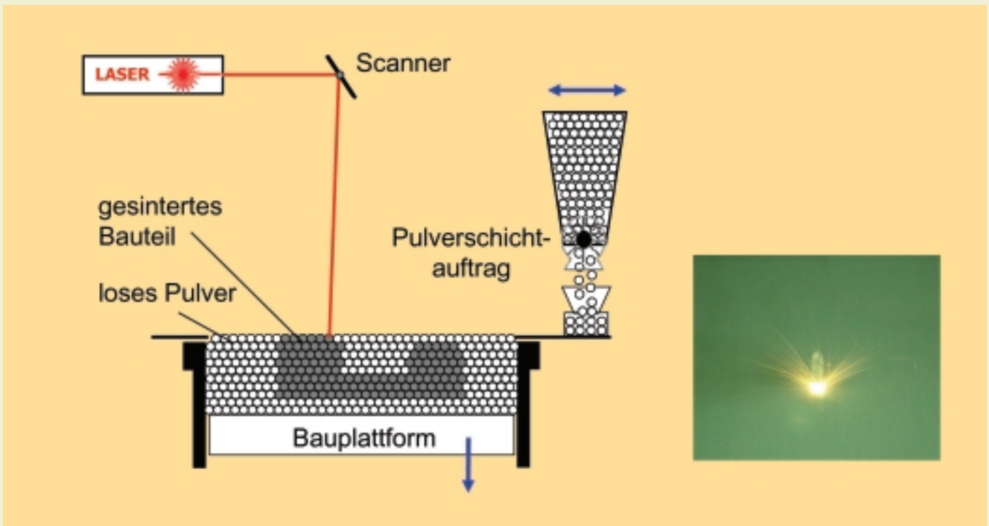
Abb. 2: Prinzip der schichtweisen (additiven) Fertigung mittels pulverbasierter Lasersinterverfahren (links) und Aufnahme des wandernden Laserfokus beim Sintern von Metallpulvern (rechts).
