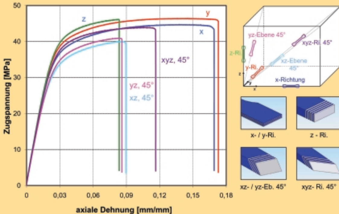
Abb. 8: Richtungsabhängigkeit der mechanischen Festigkeit von Probekörpern beim Lasersintern von Polyamid-12. Die Lage der Probekörper im Bauraum ist rechts oben skizziert. Die Belichtung erfolgt dabei jeweils in der xy-Ebene. Rechts unten ist die aus der Orientierung resultierende Schichtstruktur der Probekörper skizziert.
