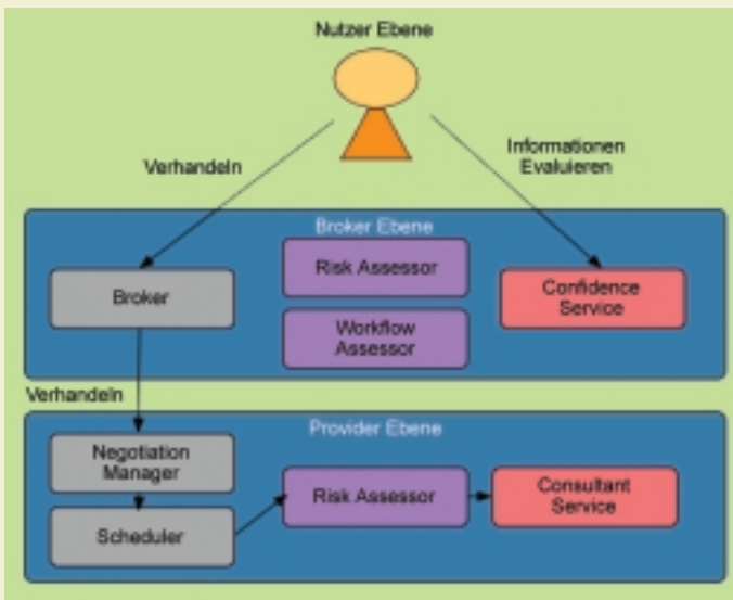
Abb. 1: Die AssessGrid Architektur.
