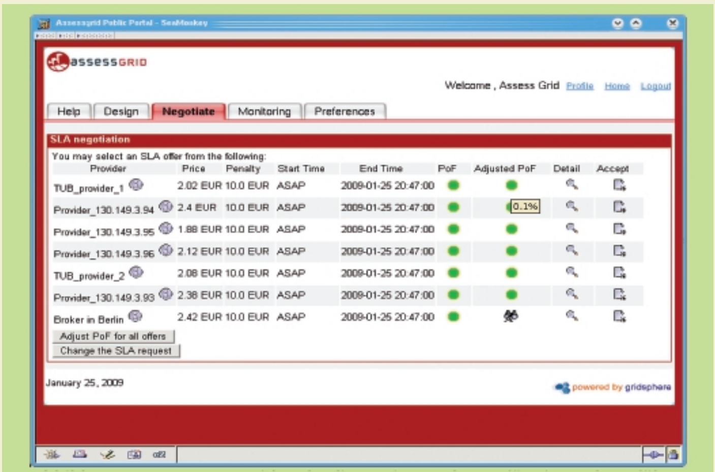
Abb. 2: Der AssessGrid Web-Client mit Angeboten für eine Jobausführung.
