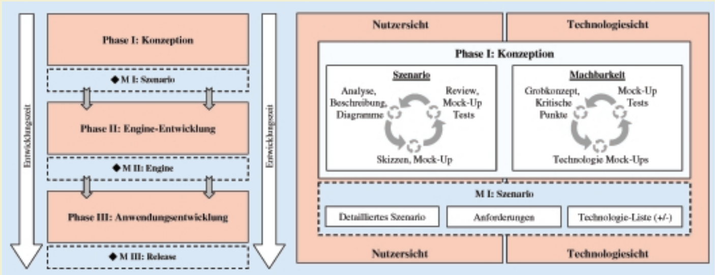
Abb. 4: Performance-orientierter Entwurfsprozess: Übersicht über die Prozessphasen (links) und Aufbau der Konzeptionsphase (rechts).
