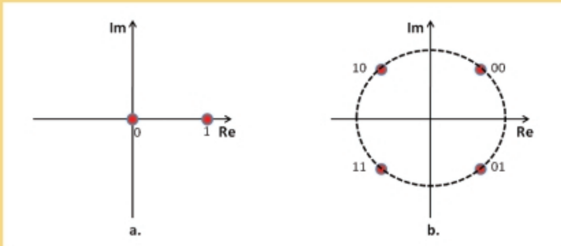
Abb. 2: Konstellaionsdiagramme für die Modulationsformate OOK (links) und QPSK (rechts). Während bei OOK nur zwischen Null und Eins unterschieden wird, gibt es bei QPSK vier verschiedene Möglichkeiten, sodass mit jedem Symbol eine zweistellige Binärzahl (00, 01, 10, 11) übertragen werden kann.
