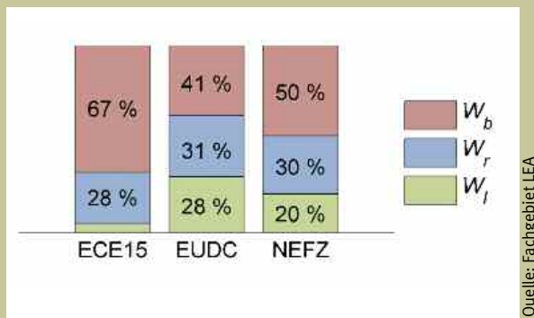
Abb. 4: Zusammensetzung des Energiebedarfs in treibenden Phasen.
