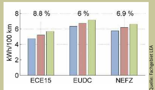
Abb. 5: Änderung des Energiebedarfs bei einer Änderung des Gewichts um 10 Prozent.
