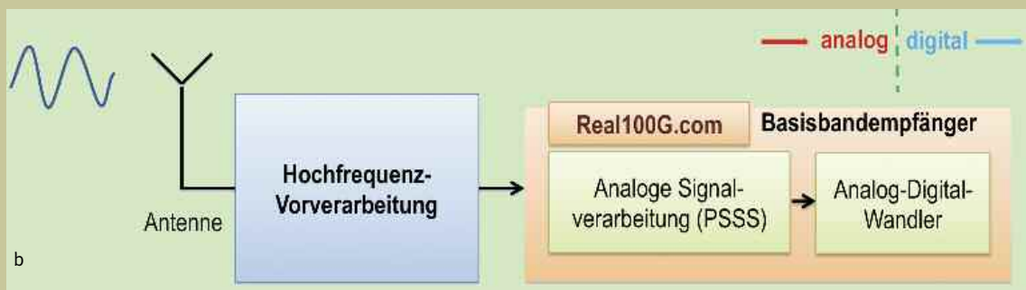
Abb. 2b: Real100G.com-Basisbandempfänger auf Basis des PSSS-Verfahrens.
