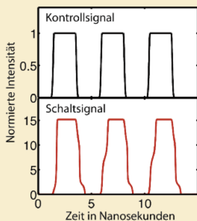
Abb. 5: Numerisch berechnete Schaltsequenz wie in [5].
