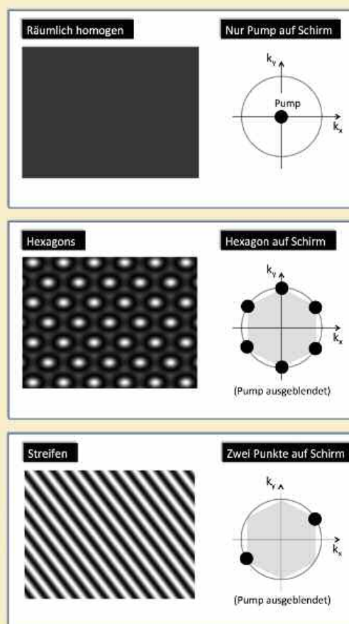
Abb. 2: Links: Räumliche Intensitätsverteilung im nichtlinearen Medium. Rechts: Zugehörige Muster auf dem Detektionsschirm.
