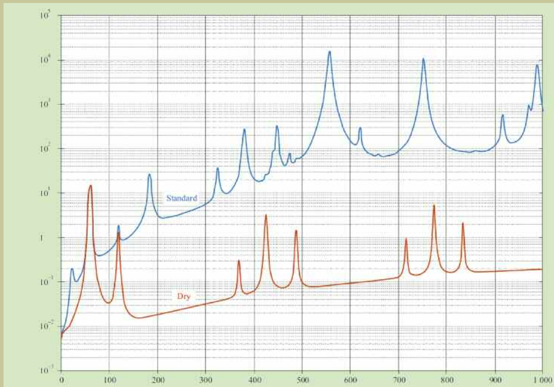
Abb. 1: Frequenzabhängige Dämpfung durch Moleküle in der Atmosphäre. [3]
