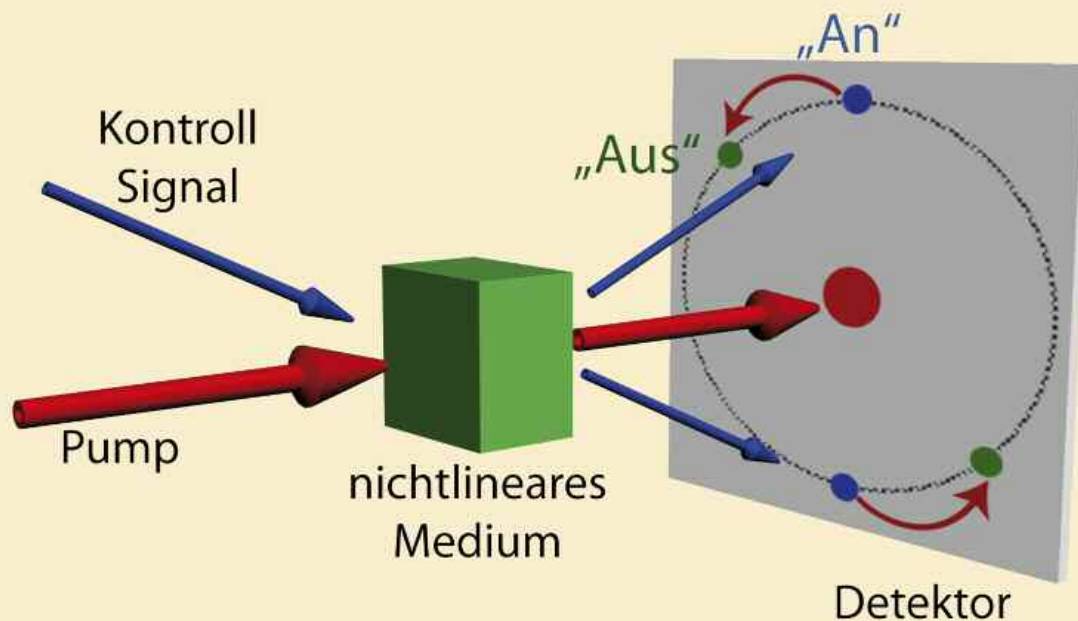
Abb. 1: Vereinfachte Darstellung eines Schaltvorgangs basierend auf optischen Mustern im nichtlinearen Medium. Die Abbildung zeigt den „An“-Zustand. Nach Abschalten des Kontrollsignals gehen das System und das detektierte Signal in den „Aus“-Zustand zurück.
