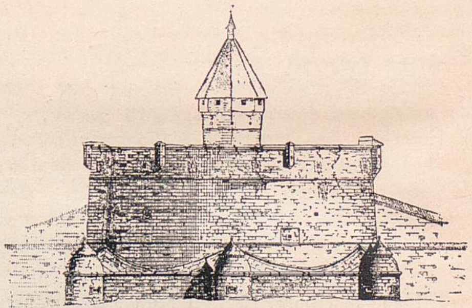
26. Schaffhausen, Außenansicht des „Unnot“. Nach J. N. Kuhn, Der Unnot in Schaffhausen. Schweizerische Bauzeitung, 1889.
