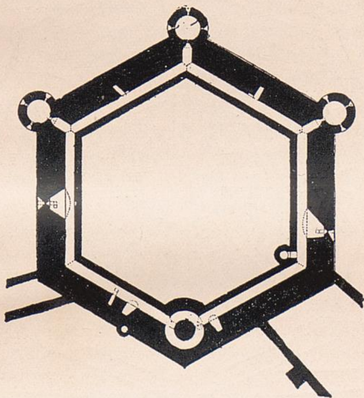
27. Schaffhausen, Grundriß des „Unnot“. Nach J. K. Kuhn, Der Unnot in Schaffhausen. Schweizerische Bauzeitung, 1889.
