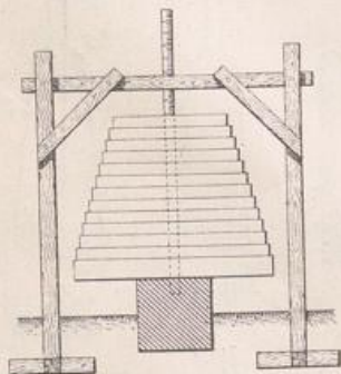
Abb. 19. Belastungsvorrichtung.
