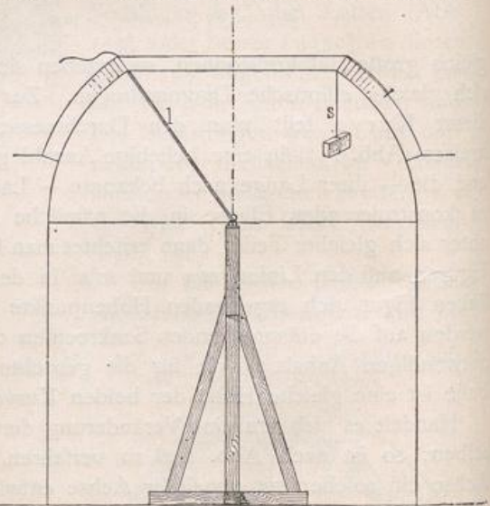
Abb. 161. Herstellung von Gewölben ohne Gerüst.
