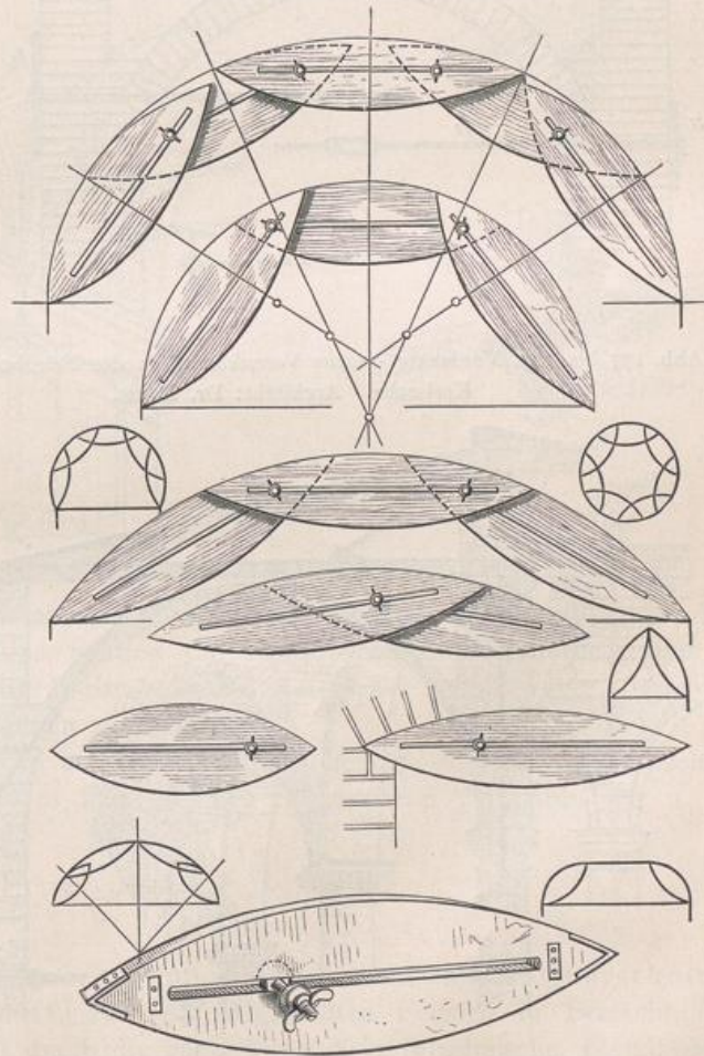
Abb. 164 bis 175. Patent-Sparbogen.
