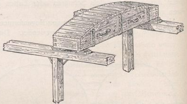
Abb. 161. Herstellung von Gewölben ohne Gerüst.
