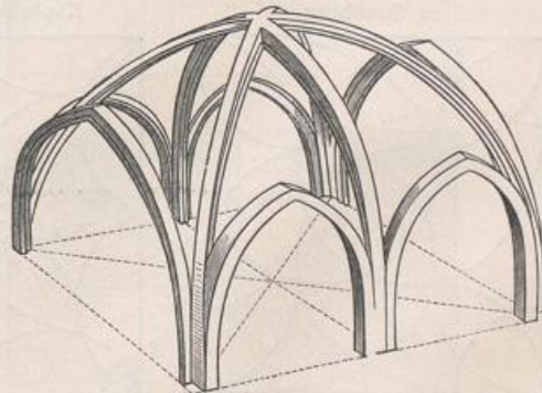
Abb. 394. Sechsteiliges Kreuzgewölbe.
