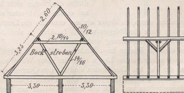
Abb. 72. Querschnitt.
