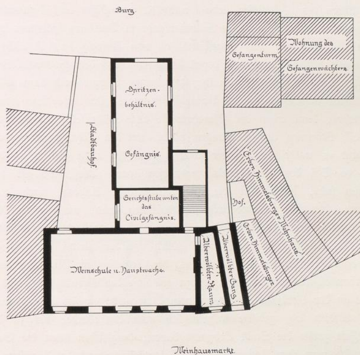
(Abbildung 2) Ältestes Rathhaus (Weinhaus). Grundriß.
