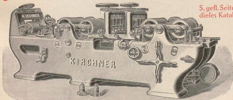
Große Rapidholzhobelmaschine: 65 m Vorschub in der Minute!
