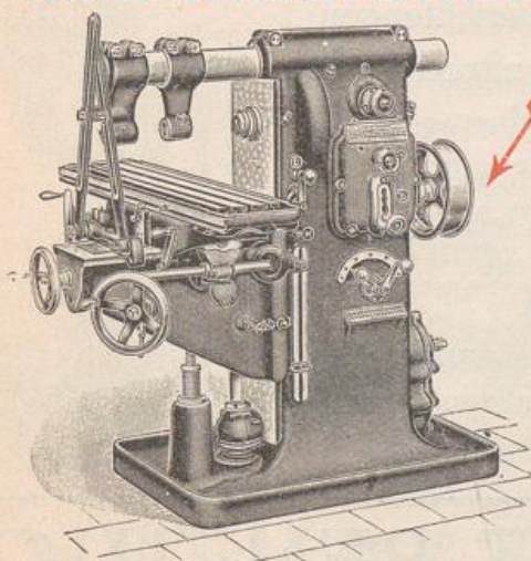
»Wanderer«-Fräsmaschine Nr. 2 mit Einzelscheibenantrieb
