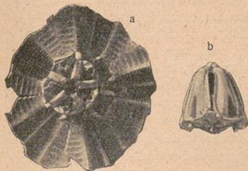
Fig. 87. Kiefergerüste ( Laterna ) eines Echiniden. a) von oben, in natürlicher Stellung, b) von der Seite.
