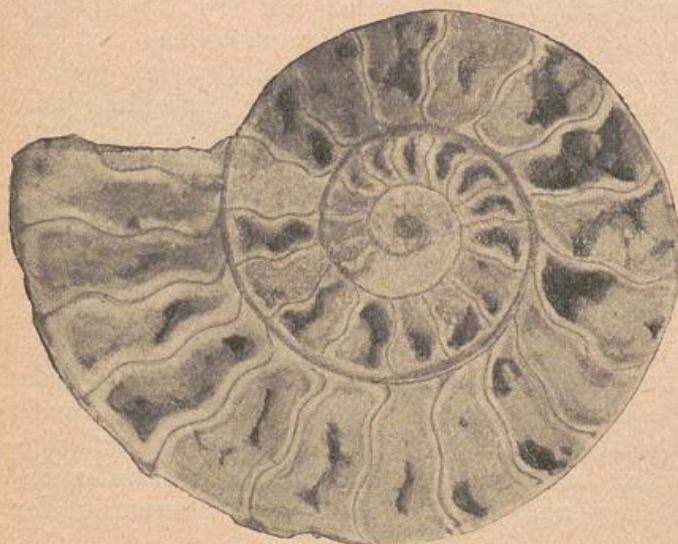
Fig. 107. Durchschnitt durch den gekammerten Teil eines Ammoniten.
