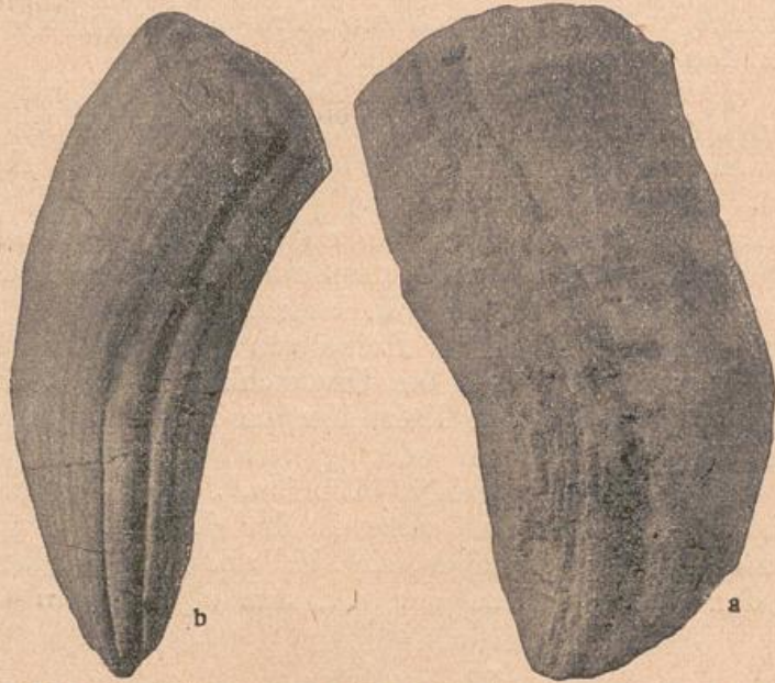
Fig. 99. Hippurites cornu-vaccinum (Goldf.) Gosaukreide \frac{1}{5} nat. Gr. a) mit Schale, b) Steinkern mit abgesprengter Deckschichte.
