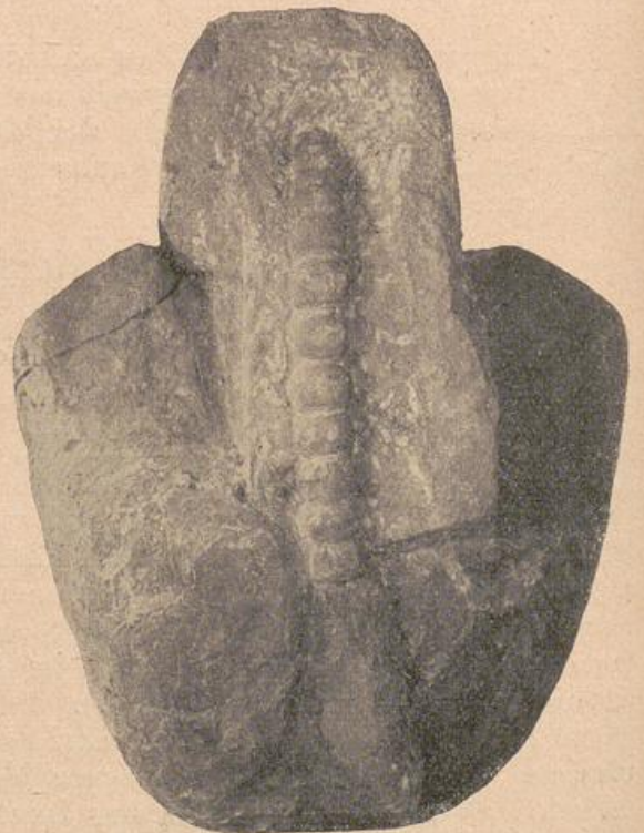
Fig. 105. Perlschnurartiger Siphon bei Nautilus bidorsatus (Schloth.).
