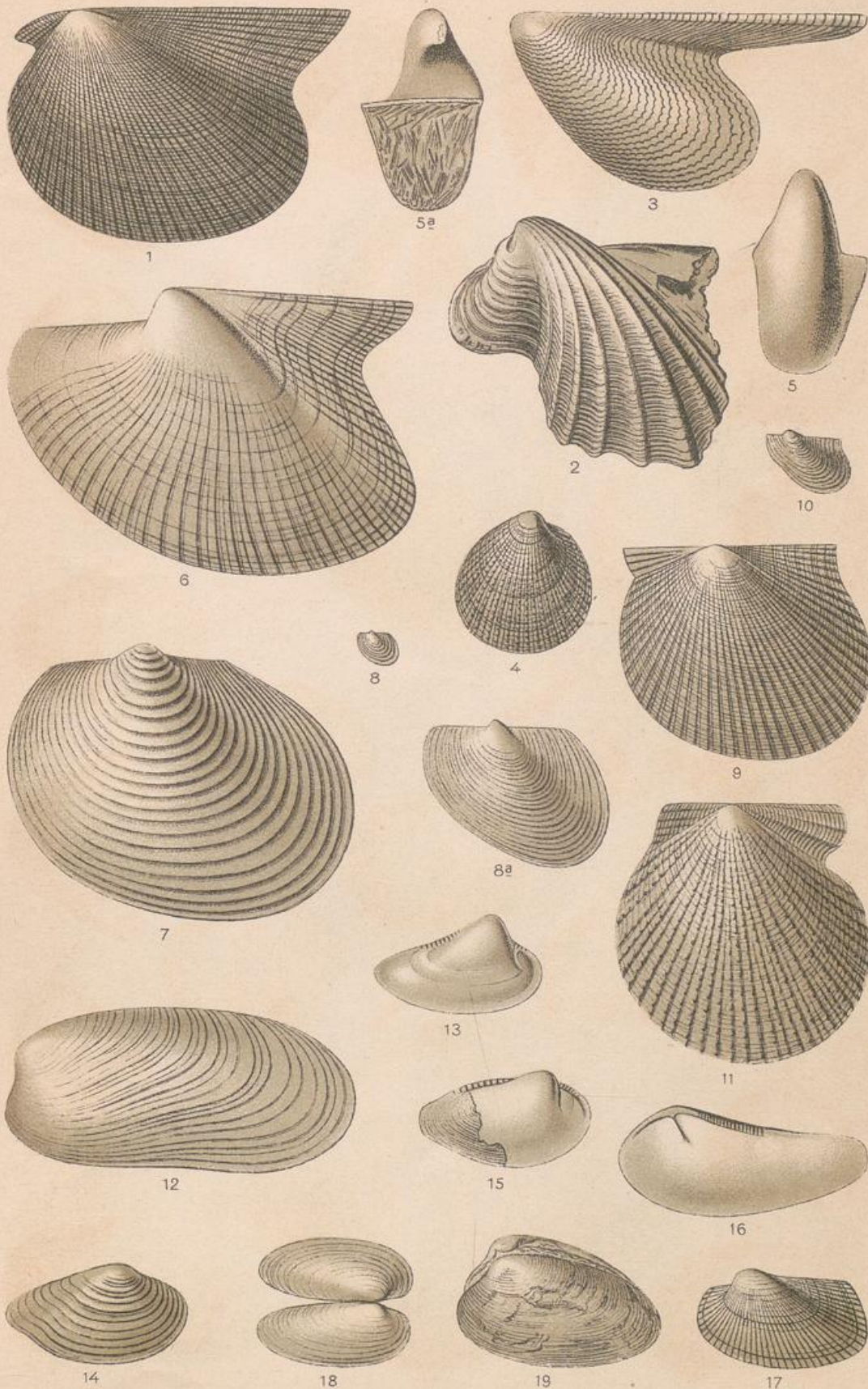
1. Pterinea lineata, 2. costata. 3. Avicula crenato-lamellosa. 4. Pseudomonotis speluncaria. 5. Kochia capuliformis. 6. Limoptera bifida. 7. Posidonomya Becheri, 8. venusta. 9. Aviculopecten papyraceum. 10. Gervillia ceratophaga. 11. Pecten grandaevus. 12. Modiomorpha lamellosa. 13. Nucula cornuta, 14. Maueri, 15. Krotonis, 16. solenoides. 17. Arca striata. 18. Anthracosia carbonaria, 19. acuta.
