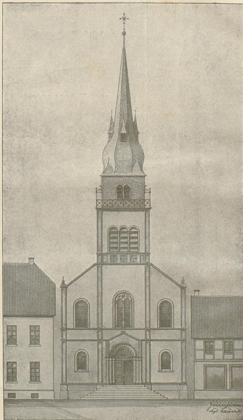
Entwurf zu einem Turmhelm für die kath. Pfarrkirche in Lemgo.
