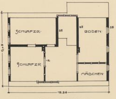
DACHGESCHOSS
