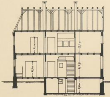
LÄNGSSCHNITT A-B
