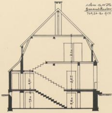
QUERSCHNITT C-D
