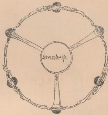
Grüchtungsgerüst mit Candelaber für 6 electr. Glühlampen
