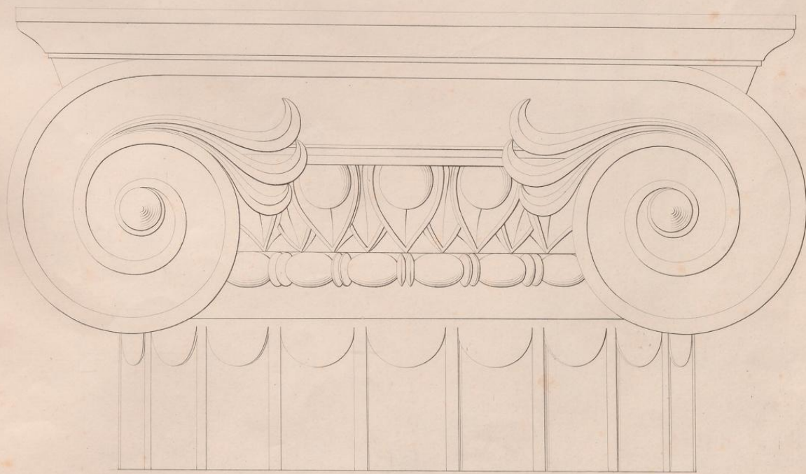
Ionisches Capital von Peperin. Stein, mit weissem Marmor überzogen, aus Pompeji.
