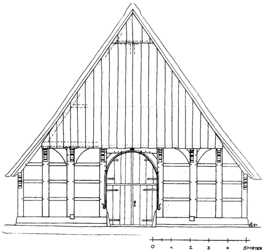
Abbildung 3: Heidenoldendorf (Stadt Detmold), ehem. Hof Mertens Nr. 12. Kötterhaus, 1558/59 (d). Vordergiebel, rekonstruierter Zustand zur Bauzeit. Aufmaß: Michels/Stiewe; Zeichnung: Verf.
