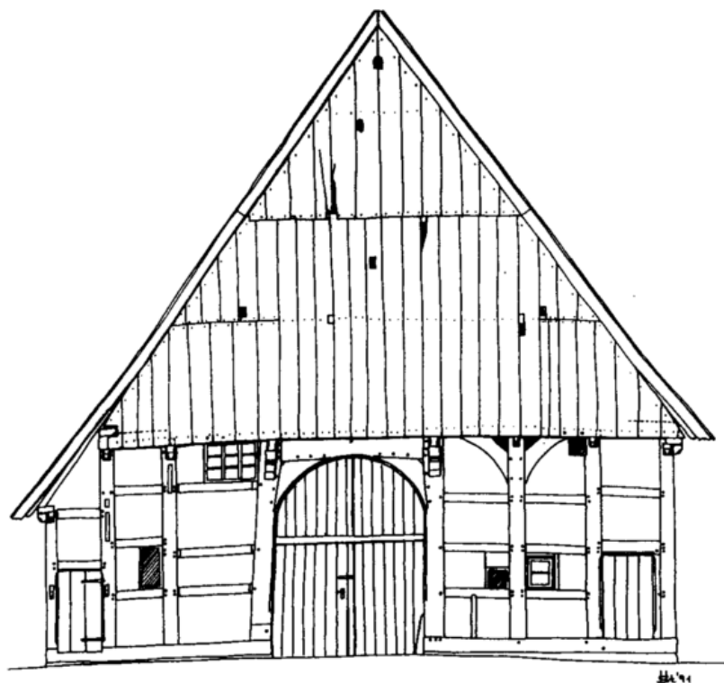
Abbildung 1: Lieme (Stadt Lemgo, Kreis Lippe), Hof Obermeyer. Ehem. Haupthaus, 1532/33 (d). Oben: Querschnitt des Zweistöckergefüges mit Blick auf die Herdwand, rekonstruierter Zustand zur Bauzeit. Unten: Vordergiebel nach Umbau zum Dreistöckerbau (Leibzuchtshaus), Zustand 1990. Aufmaß: Neumann/Sprenger; Zeichnung: Verf.
