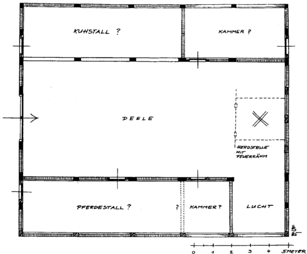
Abbildung 5. Schönemark (Stadt Detmold), ehem. Hof Klöpping Nr. 8. Bauernhaus (Großkötter), 1573 (i). Grundriss, rekonstruierter Zustand zur Bauzeit. Aufmaß und Zeichnung: Verf.
