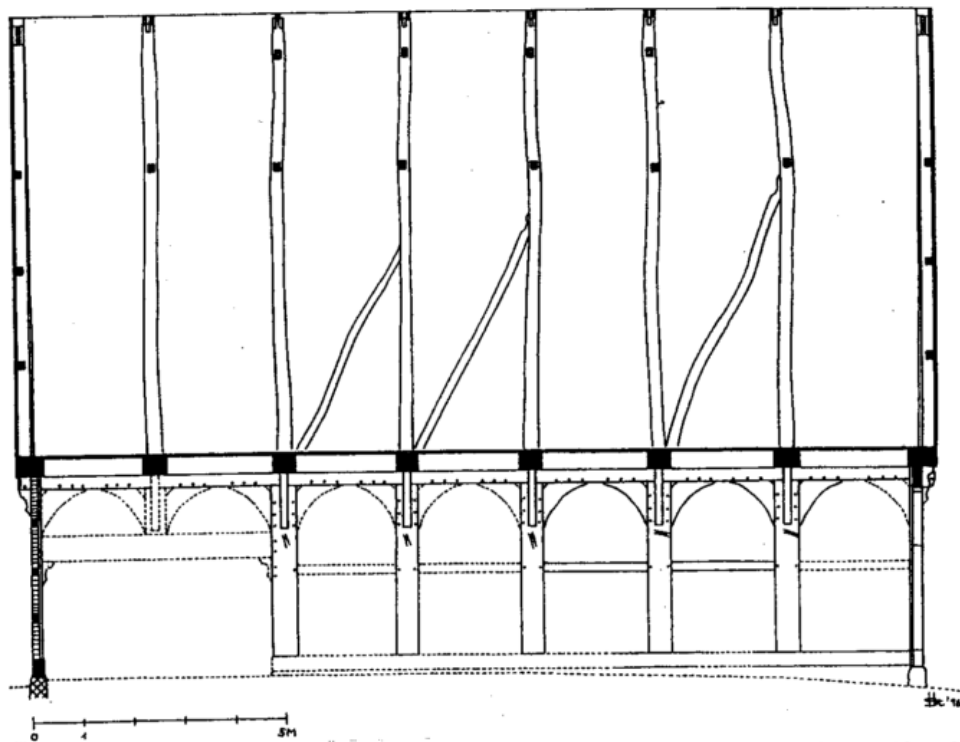
Abbildung 2: Asemissen (Gem. Leopoldshöhe, Kr. Lippe), Hof Meier zu Asemissen. Altes Meierhaus, 1555 (d). Oben: Vordergiebel, Zustand 1986. Unten: Längsschnitt mit Blick zur linken Dielenseite, rekonstruierter Zustand zur Bauzeit. Aufmaß und Zeichnung: Verf.
