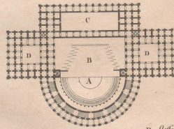
A Saal . B Bühne . C Foyer der Schauspieler . D Öffentliche Logen . Unterbau . Bedachte Auffahrt für Wagen .
