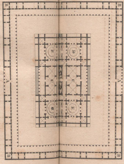
В. Црква св. Саве Г. Источна страна
