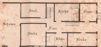
Fig. 4. Grundriß eines Fachwerkhäuses in Hörter.
