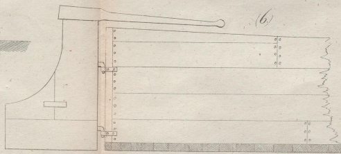
Ansicht des hinteren Theils des Schiffes
