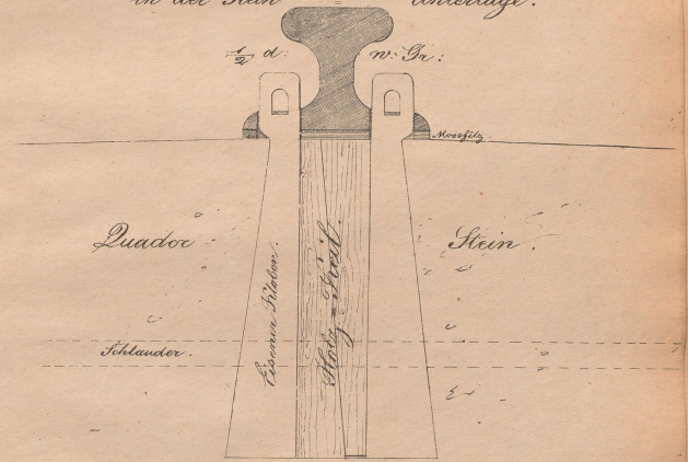
Ansicht der Schiene bei der Stoßfuge.
