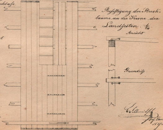
Grundriß. 1/60
