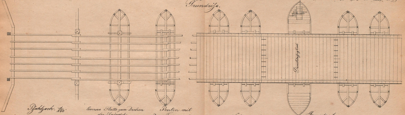
Verbindungsplatte zum Durchlaß. 1/60
