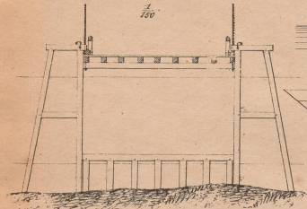
Querschnitt beim höchsten Wasserstand.
