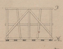
Querschnitt des Hilfsgerüsts bei F.G.
