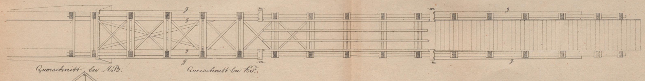
Grundriss des Daches.
