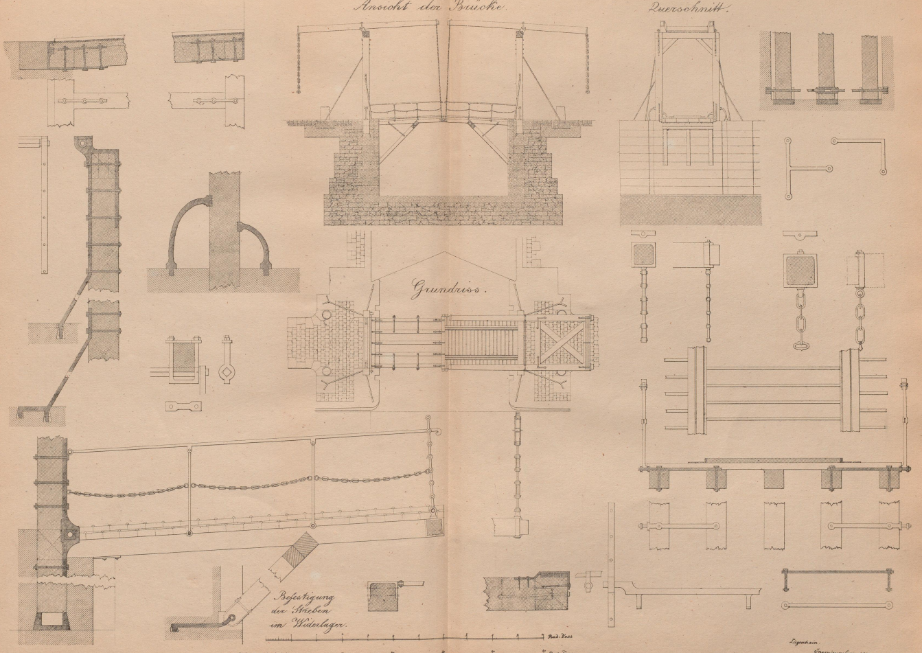
Ansicht der Brücke.
