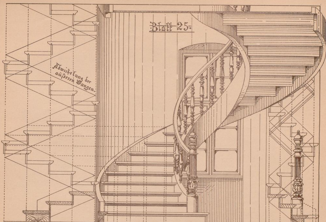
Treppe mit inneren und äußeren elliptischen Wangen.
