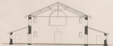
Querschnitt des Schweine-Schlachthaus
