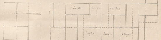
Zwei Ziegel starkes Mauerwerk.
