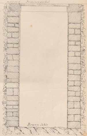
Drehschnitt.
