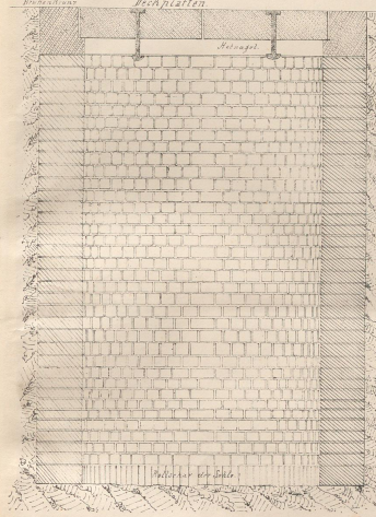
Drehschnitt.
