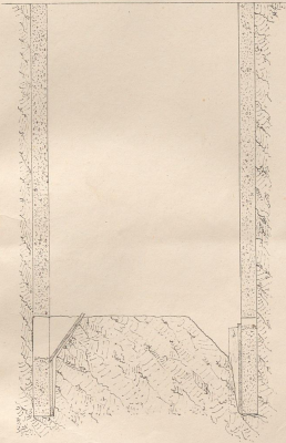
Vorgang der Untermauerung mit Betongusswandung. Drittschnitt. 2:1 u. 3:1.
