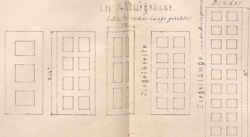
Querschnitt verschiedener Hohlziegel.
