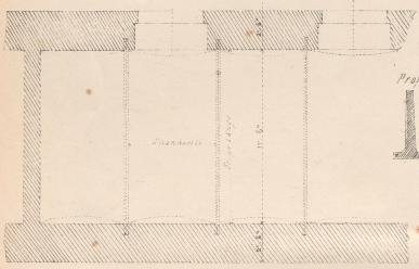
Flache Tonnen auf gusseisernen Trägern. doppelter Tafelform. Querschnitt.
