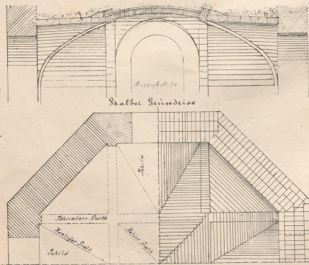
Gewölbe im Achteck mit Schilder und Gurten. Schnitt durch die Mitte.
