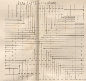
Flaches Polygonalgewölbe mit Schilder und Gurten.
