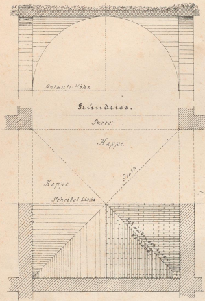
Gedrücktes Kreuzgewölbe auf Pfeilern.
