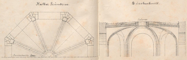
Poligonales Kreuzgewölbe mit Ziegelrippen.
