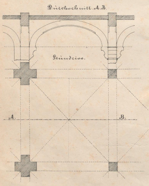
Gedrücktes Kreuzgewölbe auf Pfeilern.
