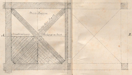
Poligonales Kreuzgewölbe mit Ziegelrippen.
