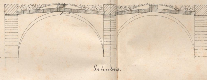
Volles Kreuzgewölbe mit Stichkappen auf vier Pfeilern. Dürchschnitt.
