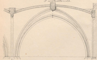
Poligonales Sterngewölbe
