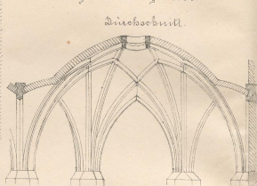
Poligonales Sterngewölbe
