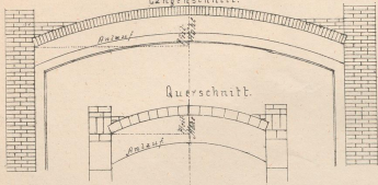
Querschnitt.
