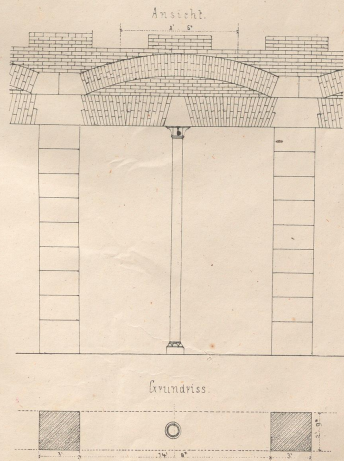
Pfeilerstellung auf gusseisene Hohl säulen. Ansicht.
