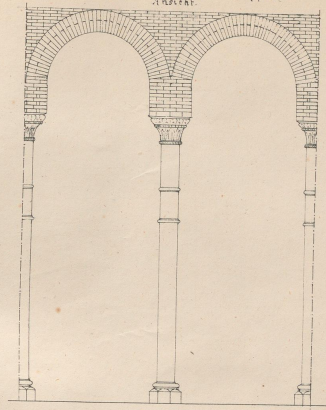
Pfeilerstellung auf gusseisene Hohl säulen. Ansicht.
