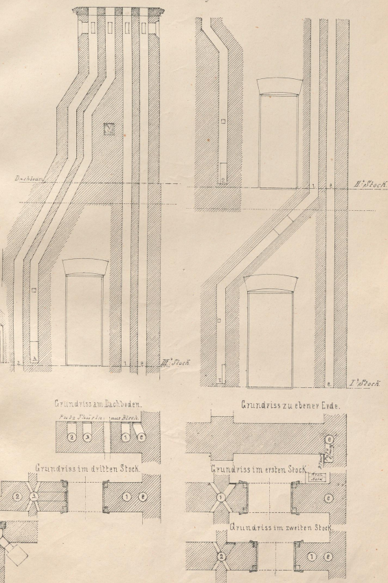
Cylinder Rauchfänge. Längenschnitte.
