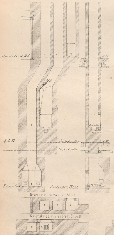
Schließbare Rauchfänge. Längenschnitt. Querschnitt.
