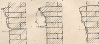
Cordon- & Stoekgesimse.
