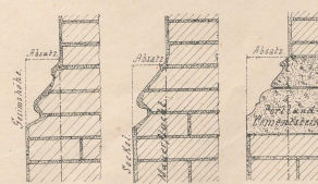
Fuss- & Soekelgesimse.
